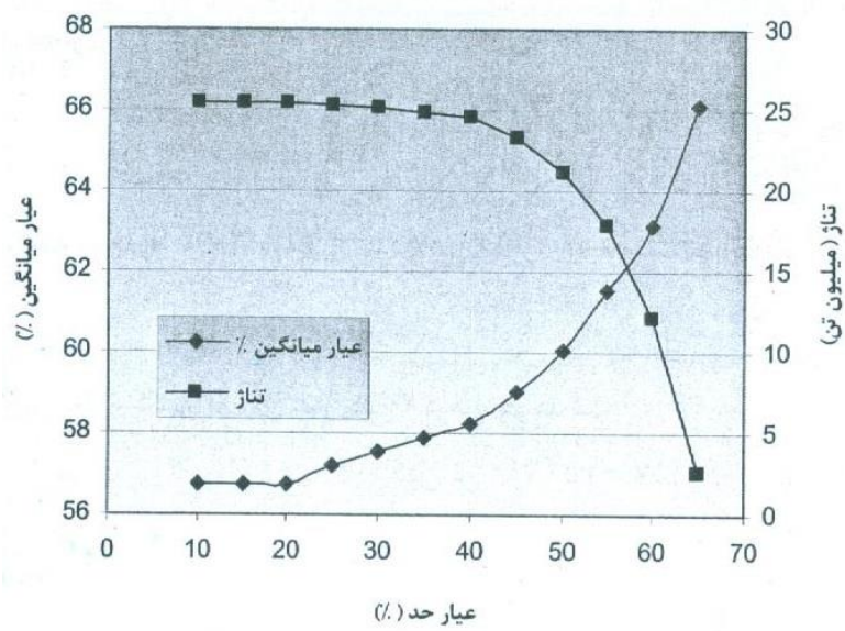
شکل ۱۱-۱- نمونه‌ای از منحنی‌های تنای-عیار برای یک کانسار سنگ آهن
